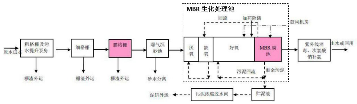
图3.2-2 污水处理工艺流程图
